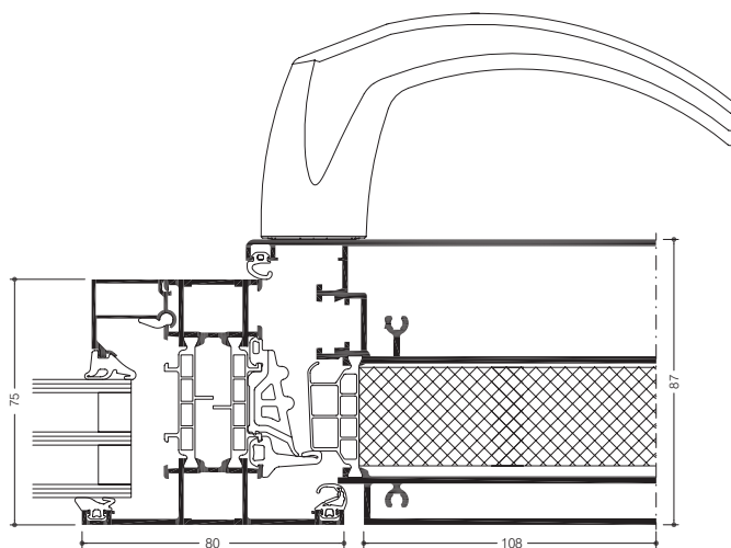
WICLINE 75 evo Ventilationslucka 180 med fönsterram
