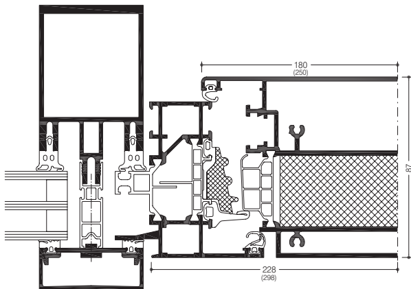
WICLINE 75 evo Ventilationslucka 250 med spännram för fasader
